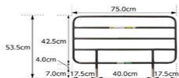
(レギュラーサイドレール PA505-75)
